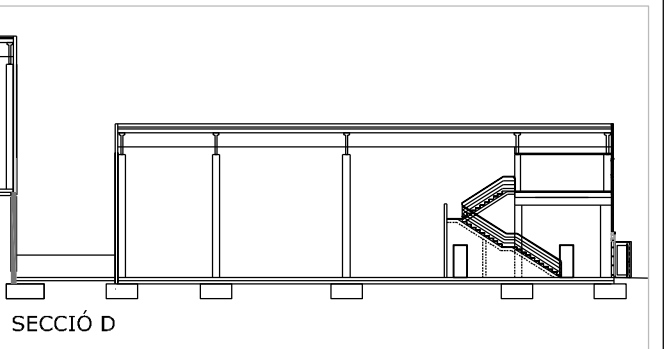
SECCIÓ LONGITUDINAL NAU
