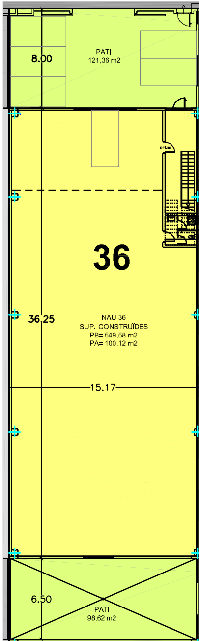
PLANTA BAIXA
