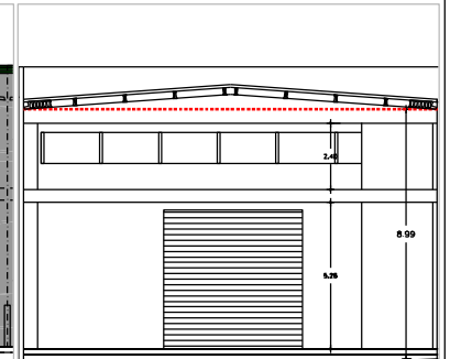
SECCIÓ TRANSVERSAL NAU
