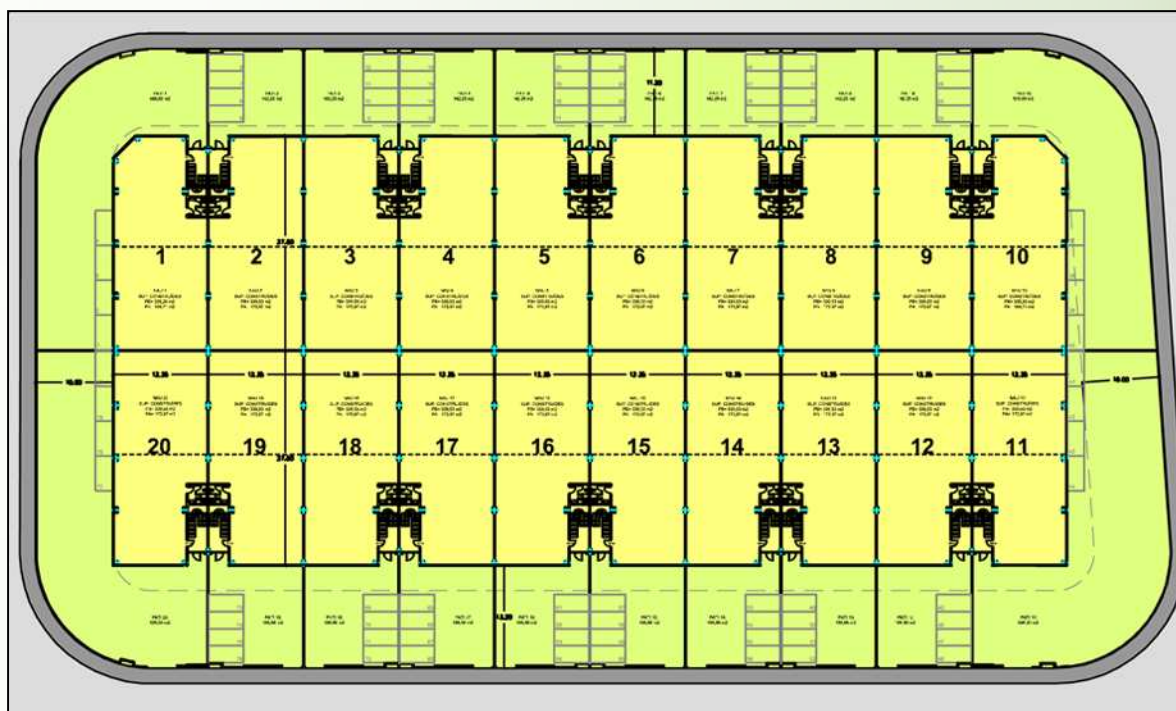
Plano de planta parcelas 20 naves
